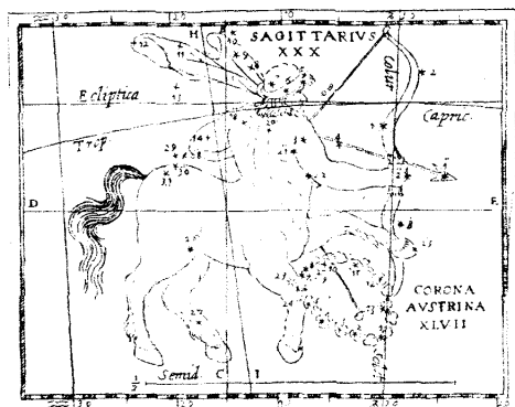
Рис. 3.17. Съзвездието Стрелец в звездна карта в книгата „Grienberdera“ [1162]. Книгохранилището на Пулковската обсерватория (Санкт Петербург). Вж. също [542], с. 46, ил. 20.
