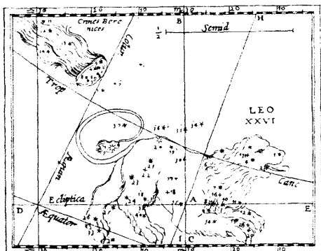
Рис. 3.15. Съзвездието Лъв в звездна карта в книгата „Grienberdera“ [1162]. Книгохранилището на Пулковската обсерватория (Санкт Петербург). Вж. също [542], с. 45, ил. 18.
