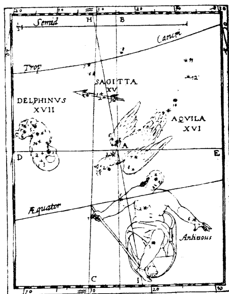
Рис. 3.18. Съзвездията Орел, Делфин и Антиной в звездна карта в книгата „Grienberdera“ (1162). Книгохранилището на Пулковската обсерватория (Санкт Петербург). Вж. също [542], с. 47, ил. 22.
