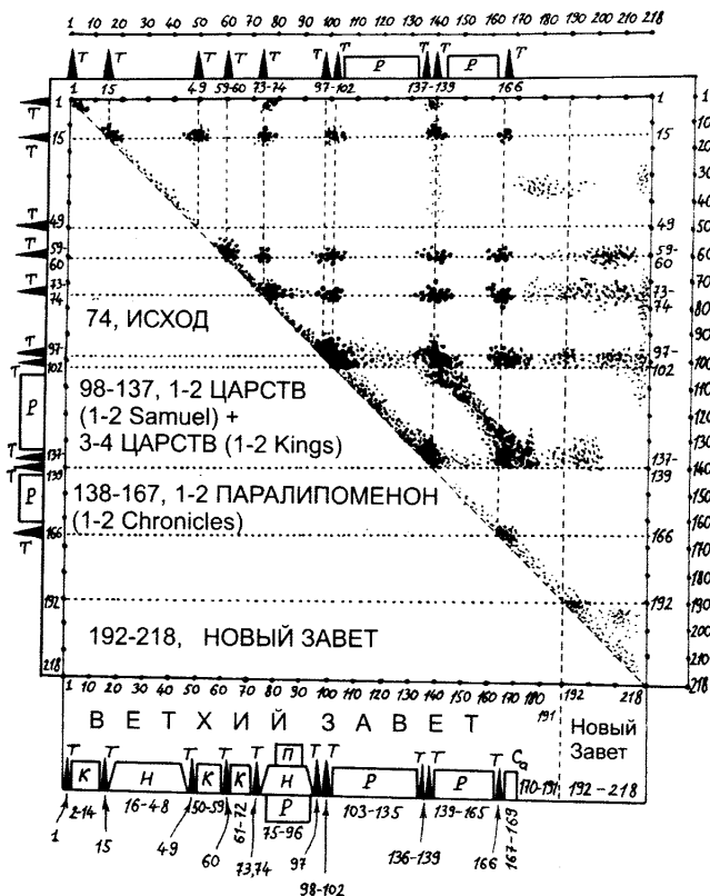
Квадратная матрица частот в Библии
